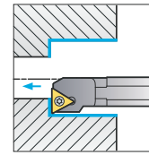
R type insert 90°
